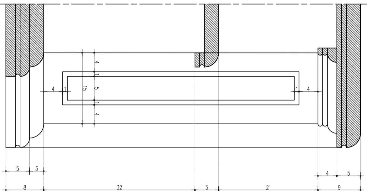
Детайл 7 Шкоф кабинет М 1:5
