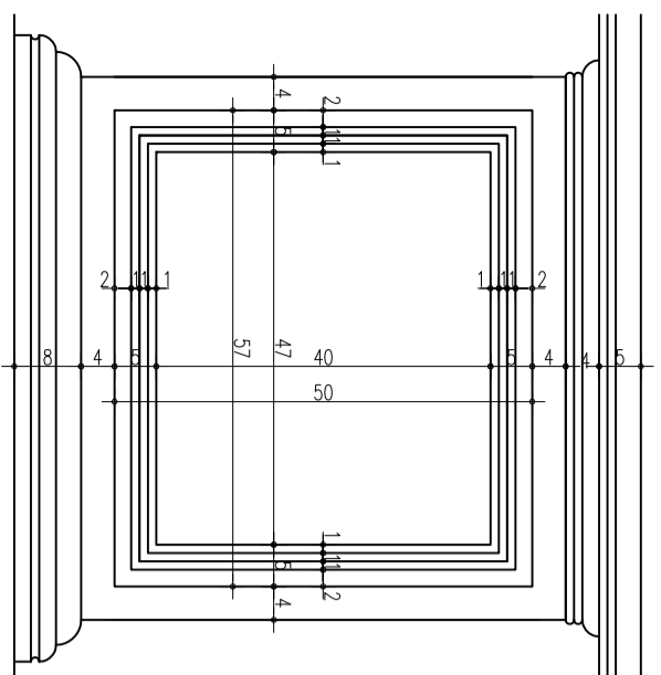
Детайл Шкоф М 1:10
