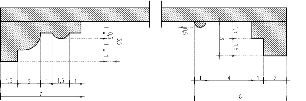
Детайл 3, М 1:10 Крок на масса Нисък шкоф Фронтент М 1:2
