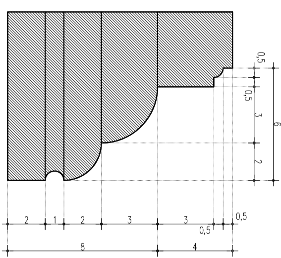
Детайл 5, 6, 7 - Фронтент Бюро и Шкоф кабинет М 1:2
