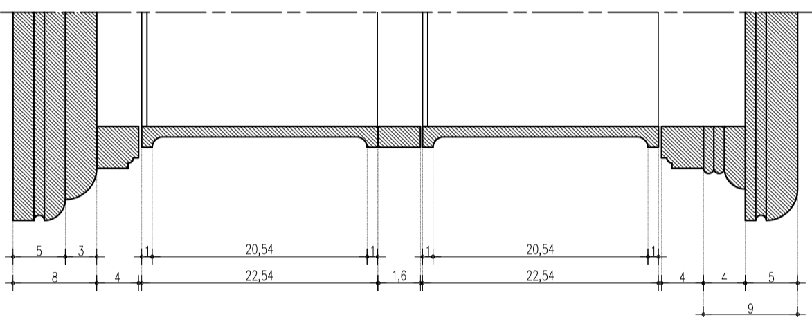
Детайл 6 Шкоф кабинет М 1:5
