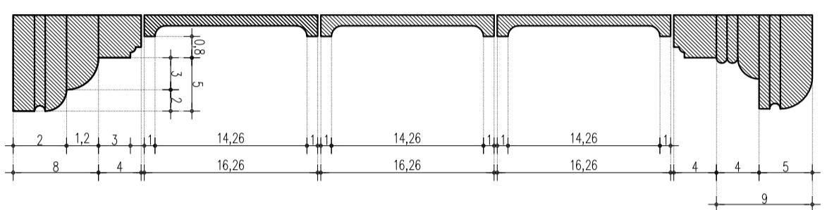
Детайл 5 Чекмакче М 1:5
